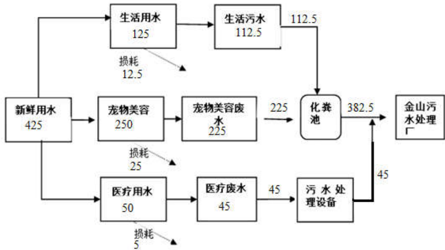
图 2.6-1 本项目水平衡图 单位: t/a
