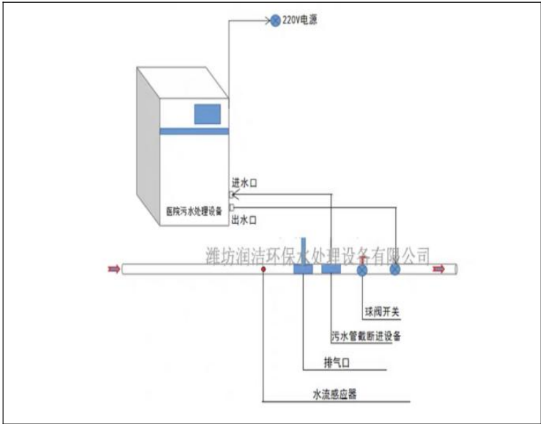
图 4-1 消毒设备接管及消毒方式
