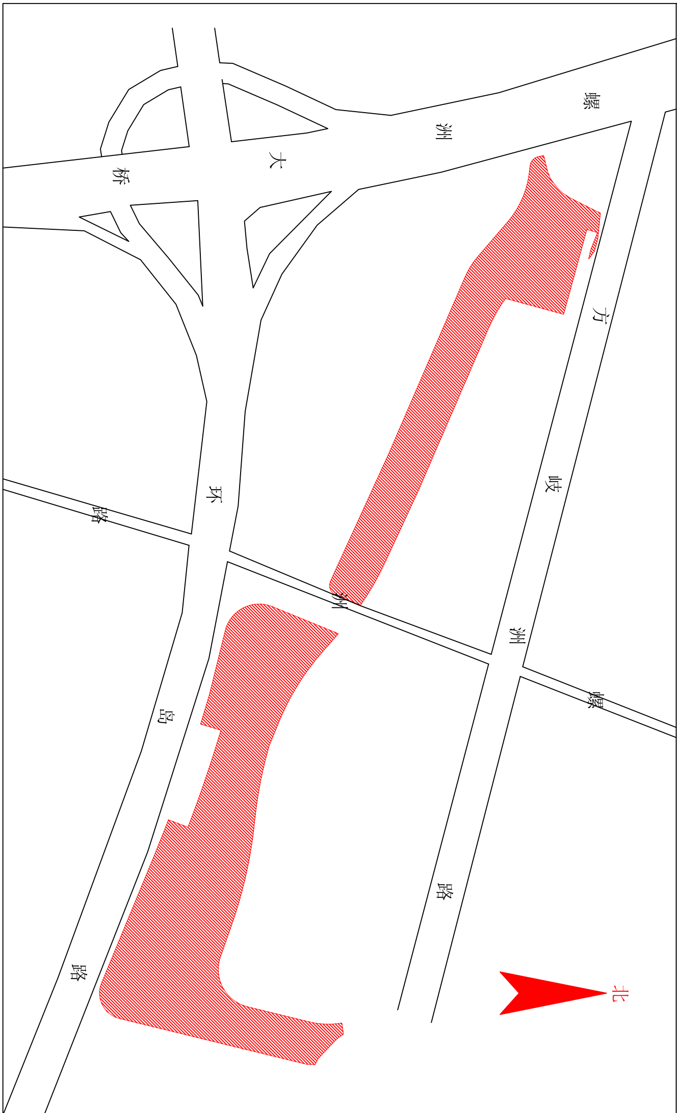
福州市螺洲四支河综合治理工程选址位置图
