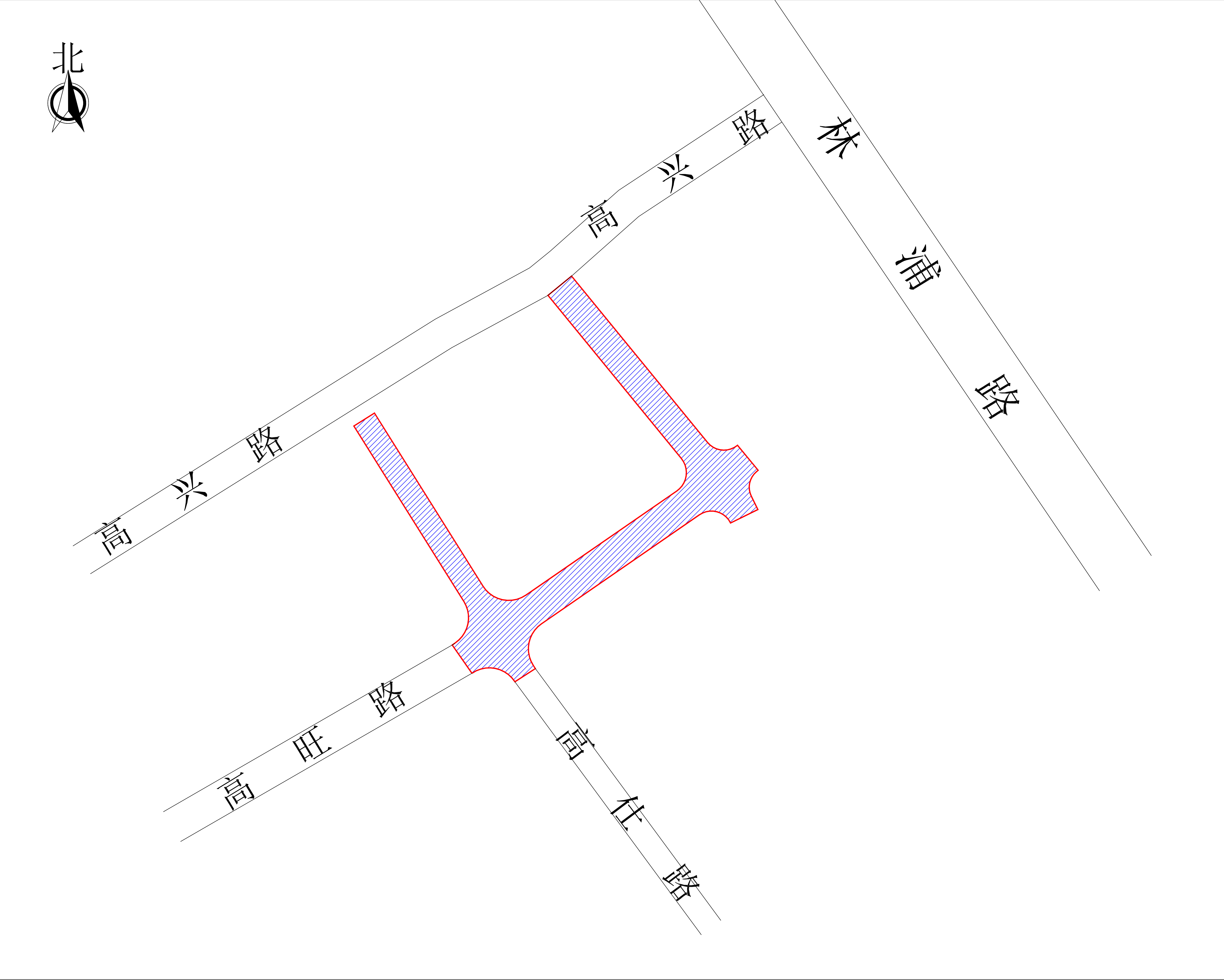
高旺路与南仕路交叉口东北侧出让地块周边配套工程项目选址位置示意图
